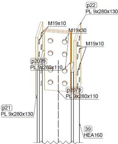
C Detalle union Columna-Columna HEA160 001 1:5
